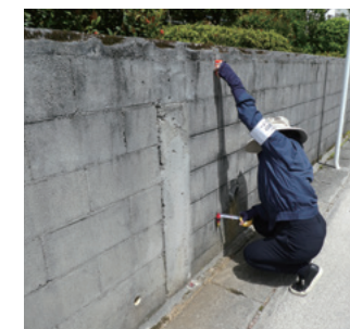
傾きの測定
