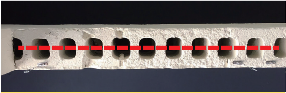
実例：改修した米軍住宅のブロック壁 鉄筋がない
