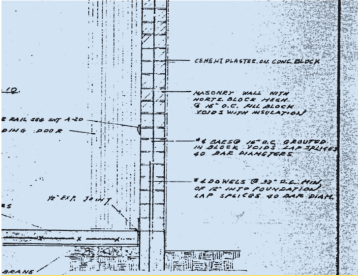
壁の設計図 1963
