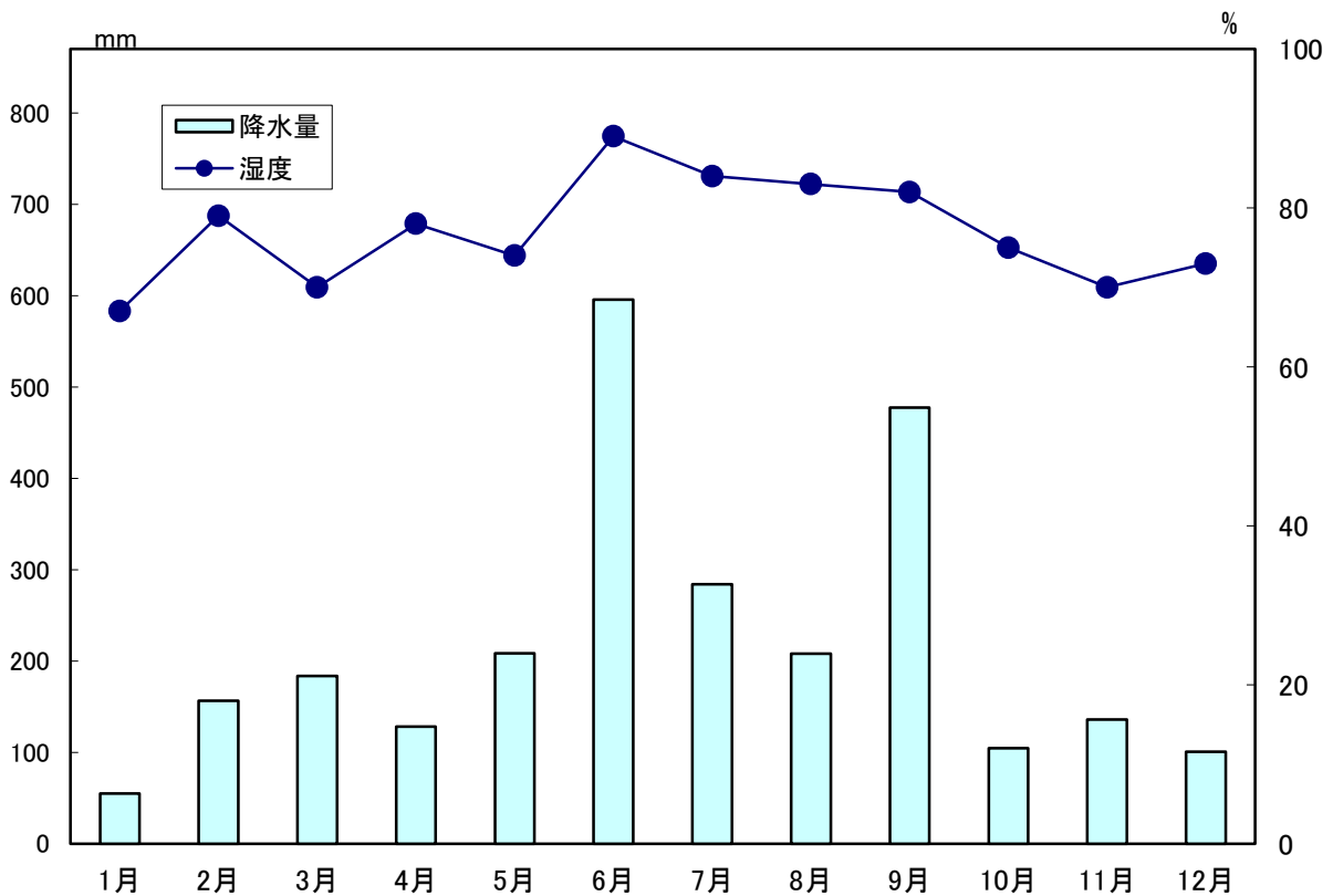
図4 月別降水量と平均湿度(令和元年)
