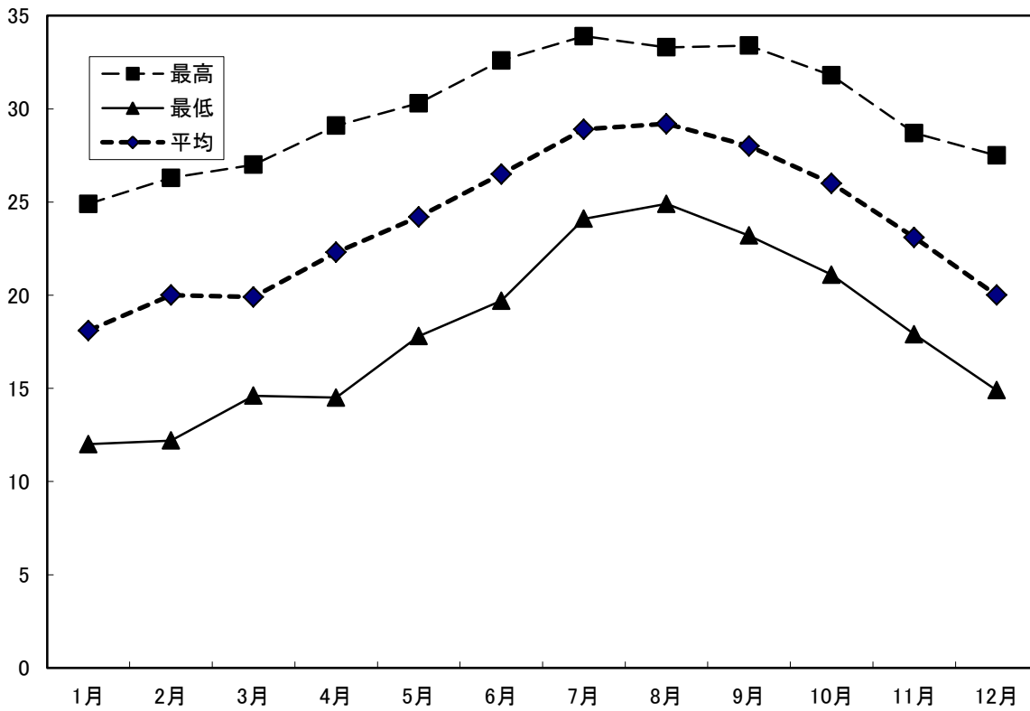
図3 月別気温の変化(令和元年)
