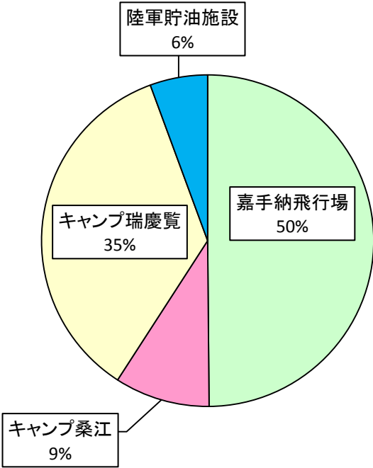
図1-2 町内における施設別米軍基地面積 (P7参照)
