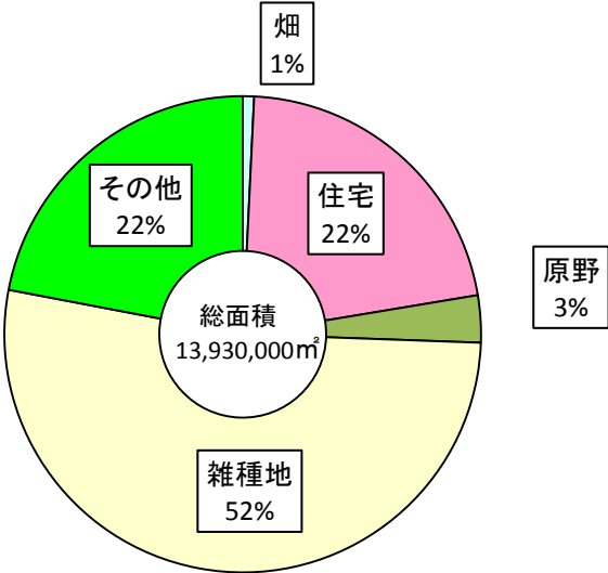
図1-1 平成31年 地目別面積(P4参照)
