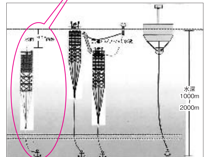
▲北谷町で採用される浮き魚礁(左側A中層型)
