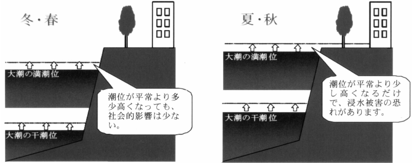
第1図 冬・春の潮位と夏・秋の潮位の比較
