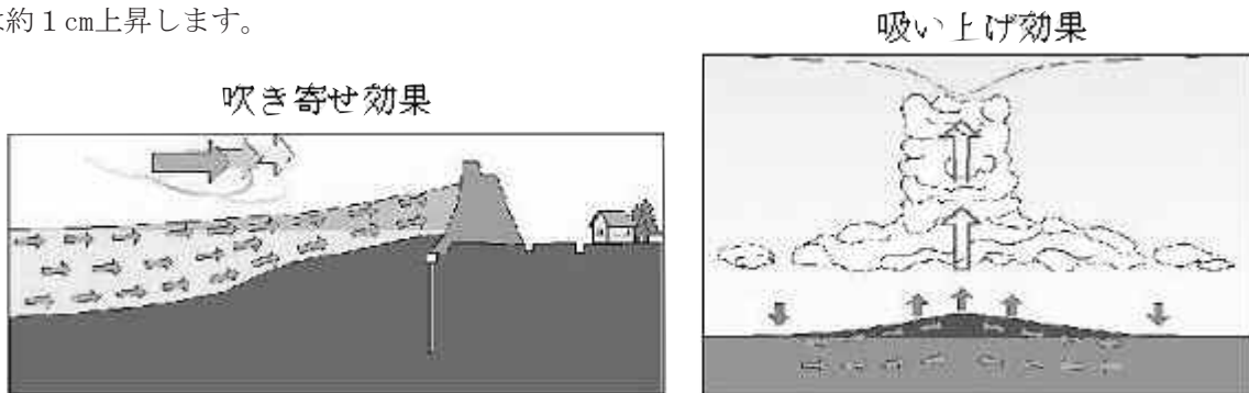
第2図 台風による高潮の発生
